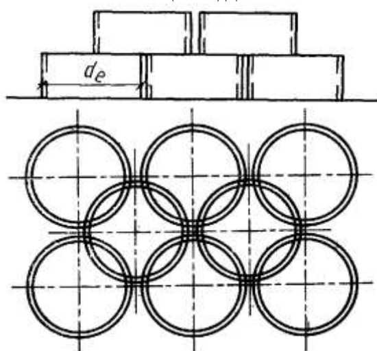
Схема складирования стеновых колец колодцев
