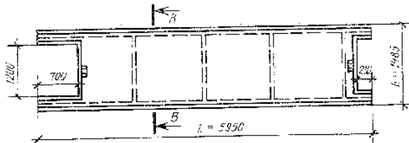
Плиты типоразмера 2П1 межколонные у торца или температурного шва здания или сооружения
