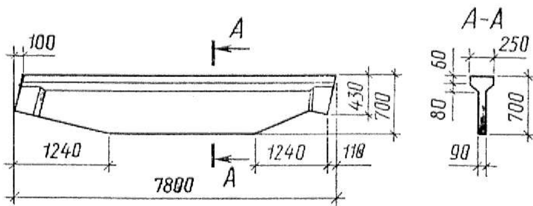
Балка типоразмера 2BCO8 (серия 1.862.1-2/88)
