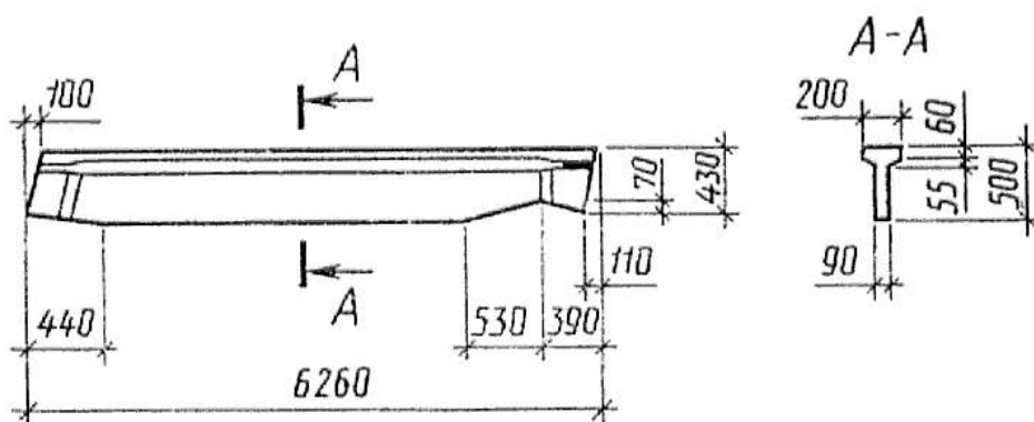
Балка типоразмера 2BCO6 (серия 1.862.1-2/88)
